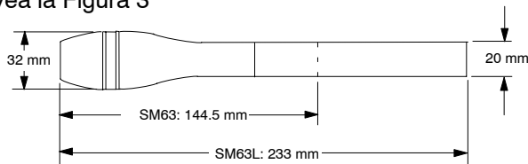
DIMENSIONES GENERALES FIGURA 3
